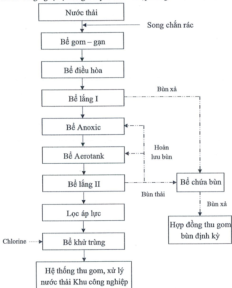
Hình 4. Sơ đồ công nghệ hệ thống xử lý nước thải tập trung tại Cơ sở
